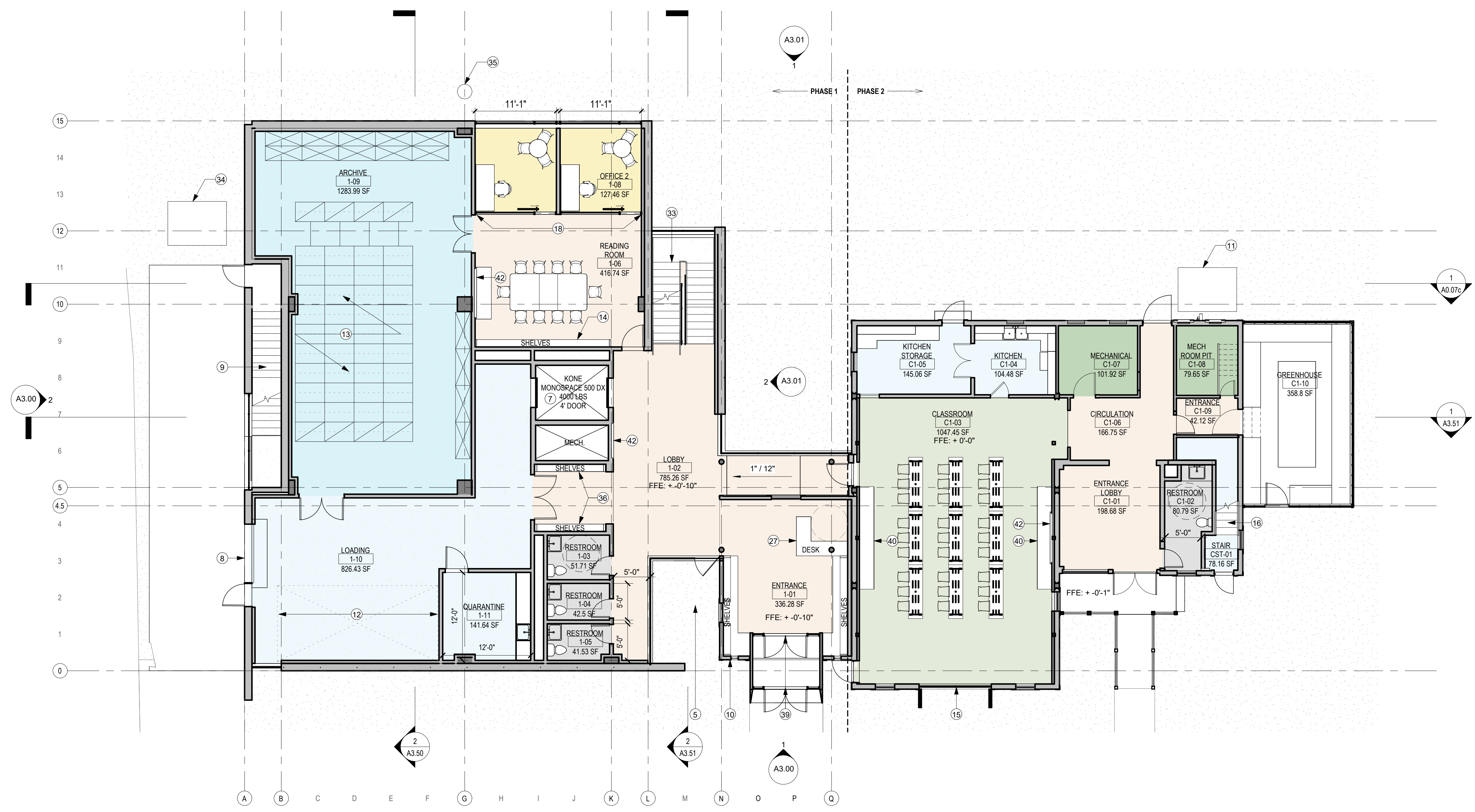
1 | Level 1 Plan SCALE: 1/8" = 1'-0"
