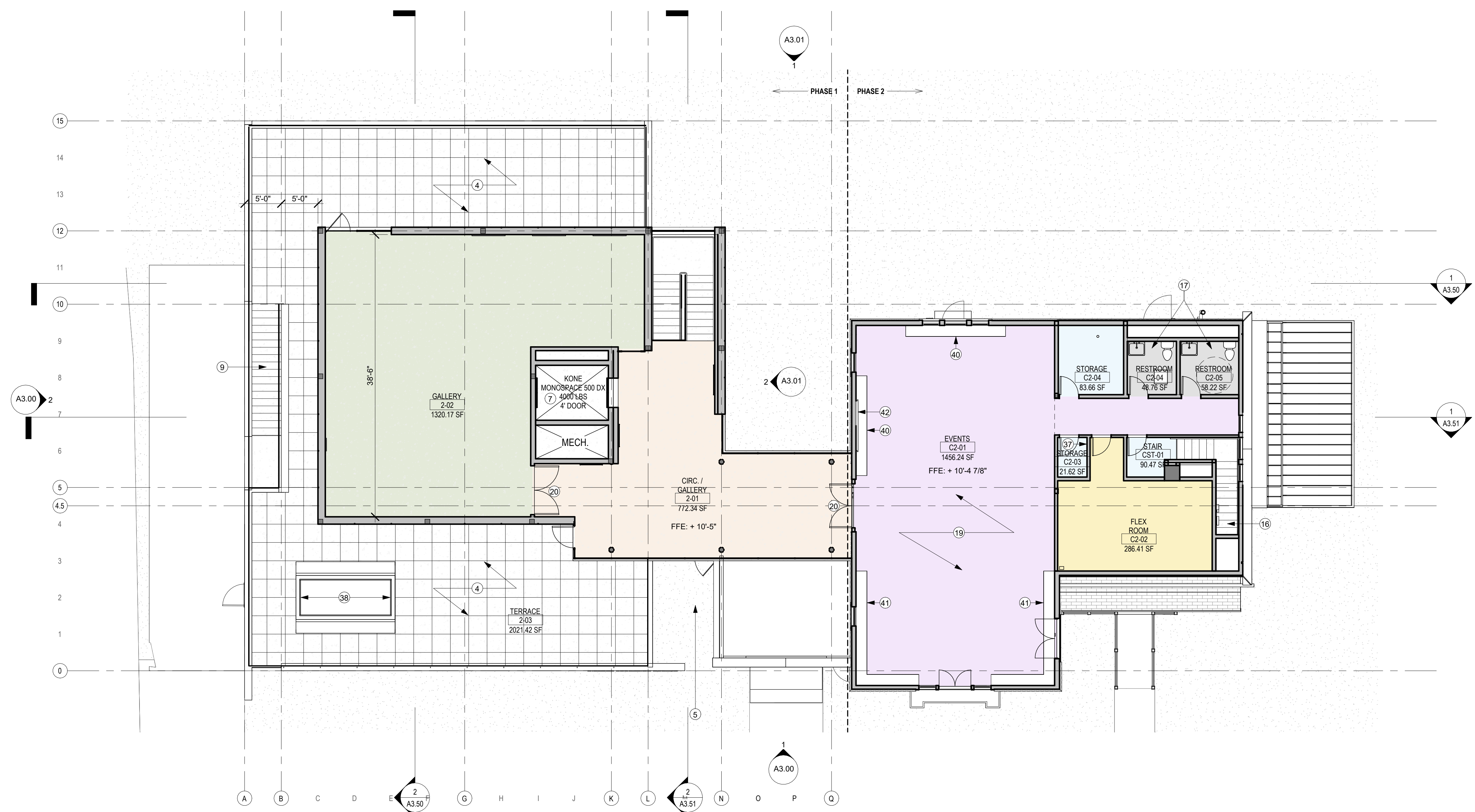
1 | Level 2 Plan SCALE: 1/8" = 1'-0"
